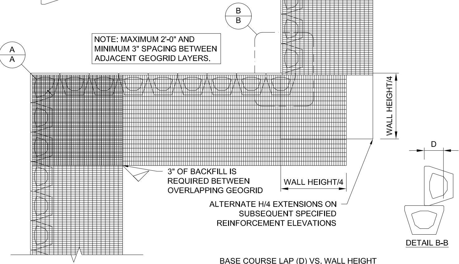
BASE COURSE LAP (D) VS. WALL HEIGHT
